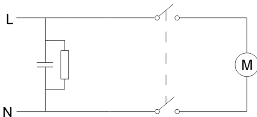
Schematic Diagram - Schaltplan - Schéma électrique - Bedringschema - Diagrama esquemático - Schema apparecchio - Esquema eléctrico
